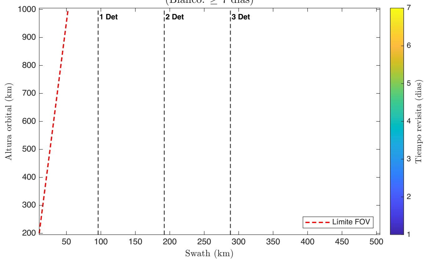
Tiempo Revisita - 1 Satelite(s); 1 Telescopio(s): Korsch; Detector 1 (Blanco: \geq 7 dias)
